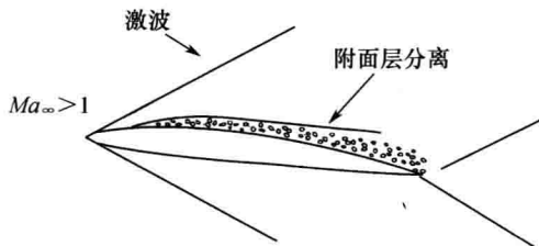
图 1.1.2 激波引起阻力的示意图
