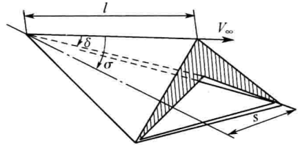
图 1.2.5 一种 V 形乘波机翼方案
