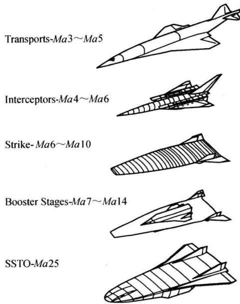
图 1.2.9 高超声速飞机的的气动布局特征
