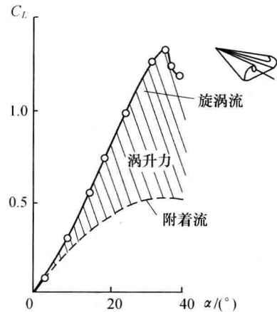
图 1.3.2 细长机翼的涡升力
