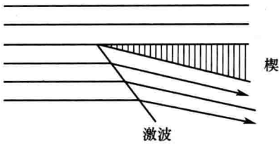
图 1.2.4 流经二维的超声速流动
