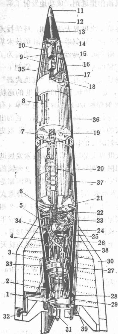
图 0.3 V-2弹道式导弹结构图
