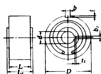
CKA型单向楔块式超越离合器基本参数和主要尺寸（其它型号省略）
