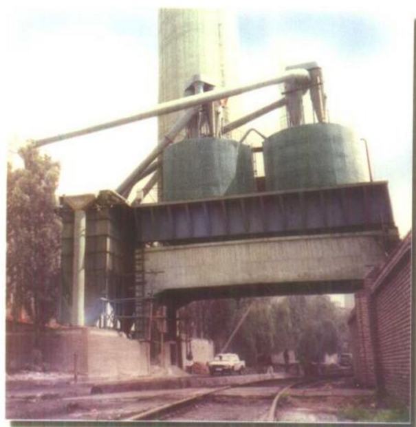
神头电厂粉煤灰气力输送及分选系统
