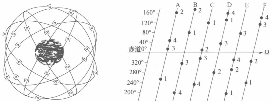
图 1-1 GPS 卫星星座及其平面投影
