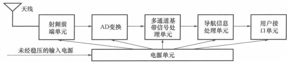
图 1-4 GPS 接收机基本构成
