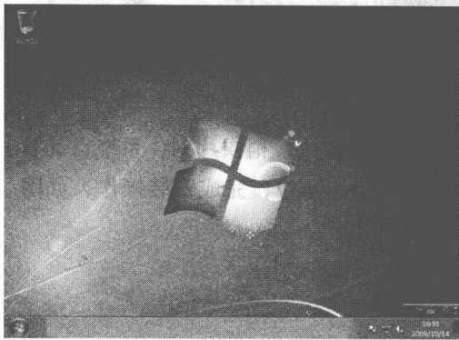
图1-28 Windows 7桌面
