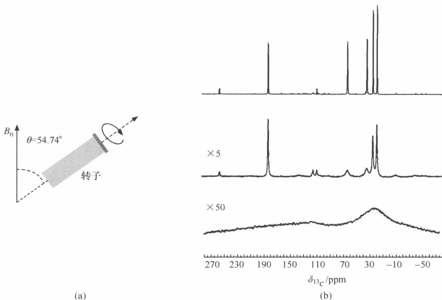
图 1-1 (a)魔角旋转示意图;(b) [^{13}\text{C}, ^{15}\text{N}] 标记缬氨酸静态固体 ^{13}\text{C} MAS NMR 谱(下)、魔角旋转转速 11kHz 下 ^{13}\text{C} MAS NMR 谱(中)以及对 ^1\text{H} 核进行 SPINAL 异核去耦下的 ^{13}\text{C} MAS NMR 谱(上)
