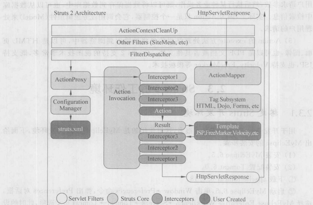
图 2-3 Struts 2 的框架结构
