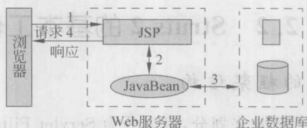
图 2-1 Model1 的流程图
