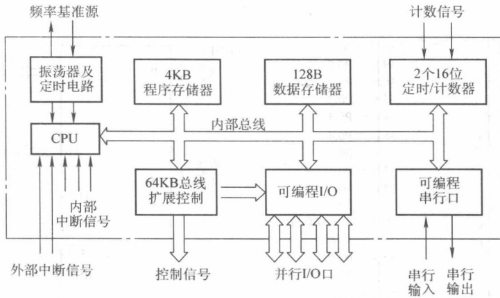
图 2-2 8051 结构框图
