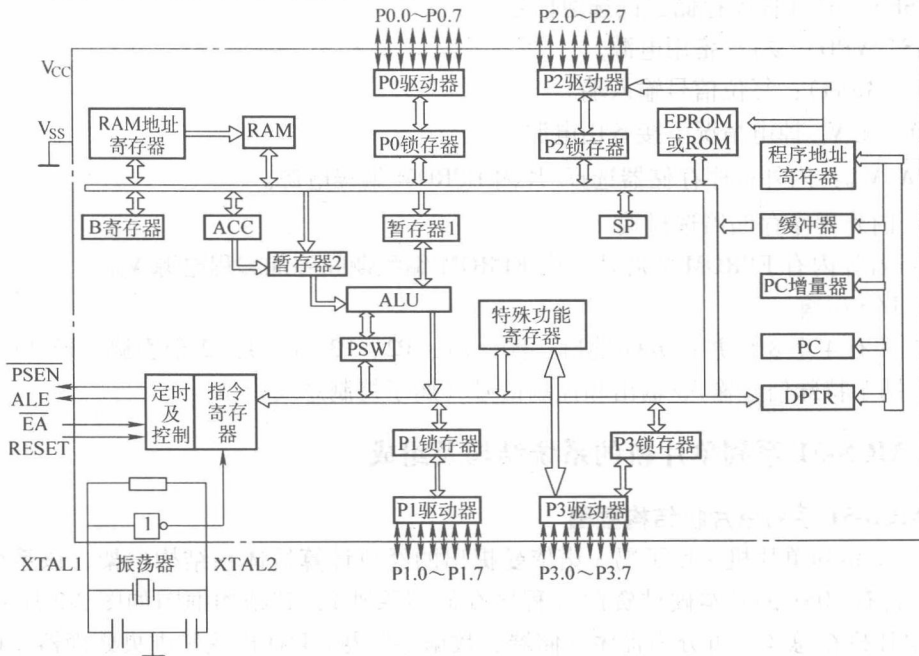
图 2-3 MCS-51 系列单片机芯片的内部结构
