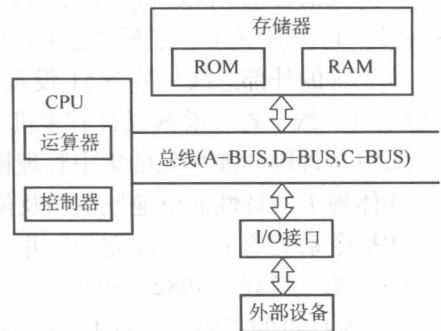
图 1-1 微型计算机基本组成框图
