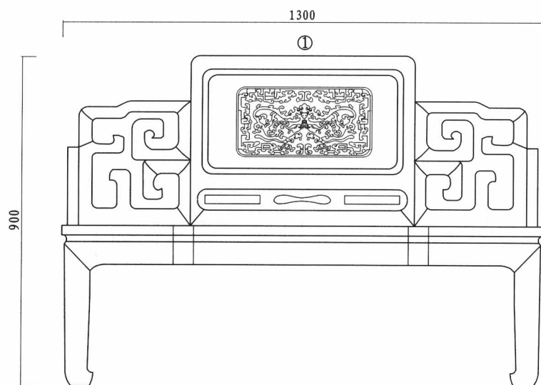
主视图 front view
