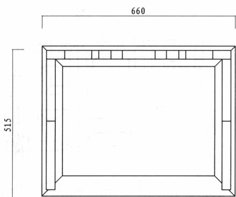
俯视图 top view
