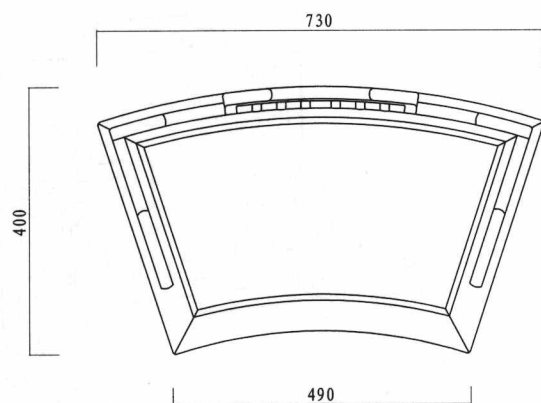
俯视图 top view
