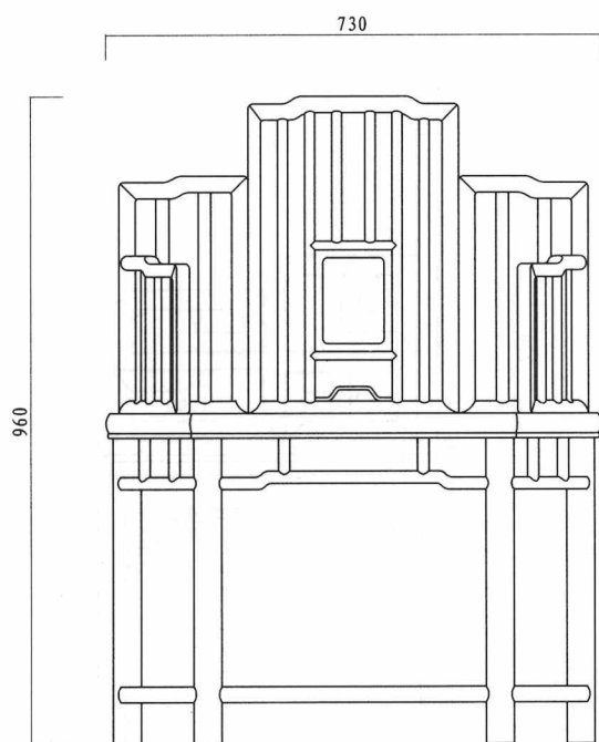
主视图 front view
