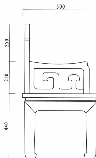
左视图 left view
