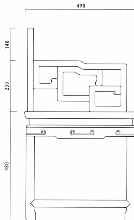
左视图 left view
