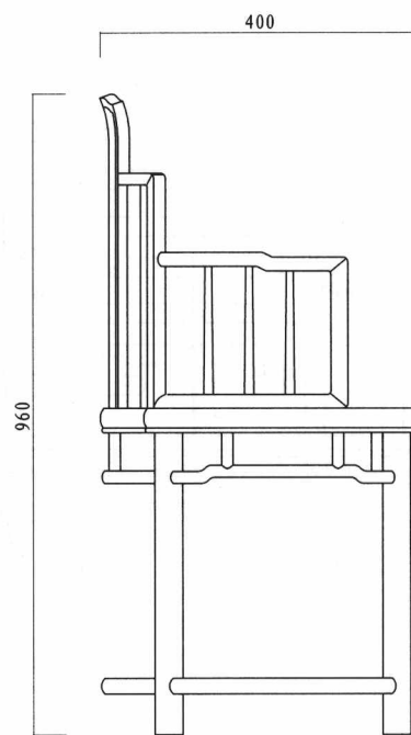
左视图 left view
