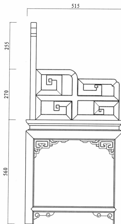
左视图 left view
