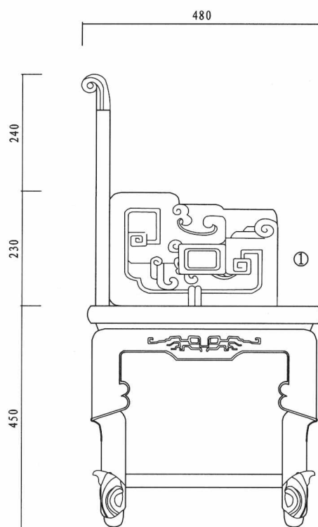
左视图 left view
