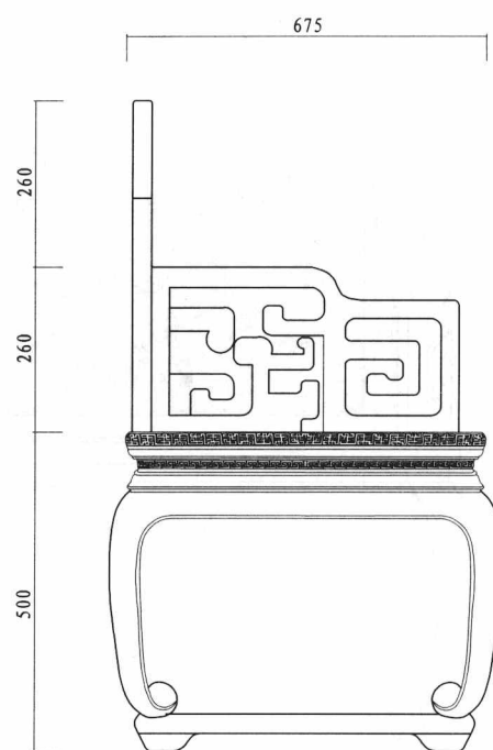
左视图 left view
