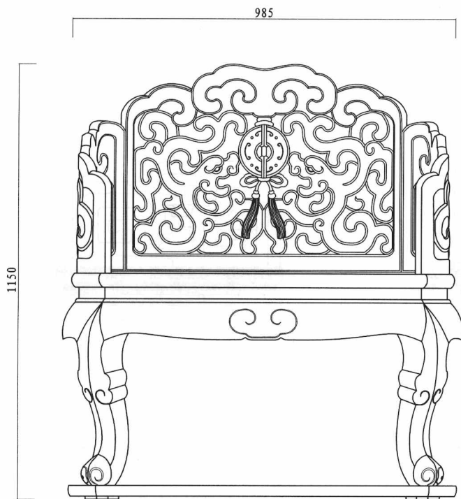
主视图 front view
