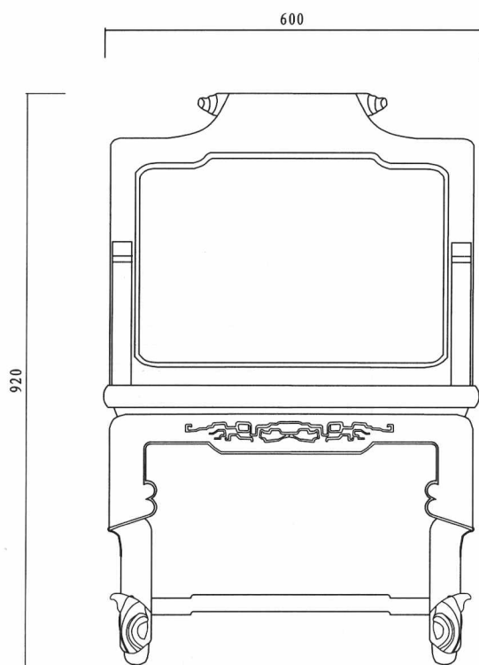
主视图 front view
