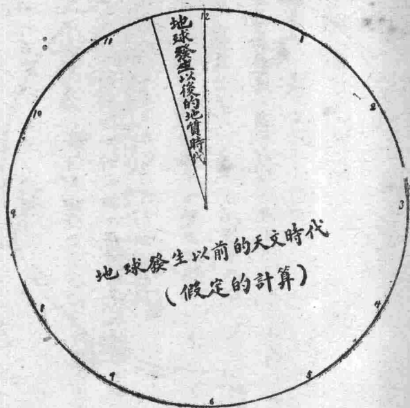
第一圖 天文時代和地質時代
