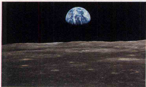
从月球上看,地球白天的一面在夜空中显得很壮观,因为月球上没有大气,所以视线不会受到阻碍。
