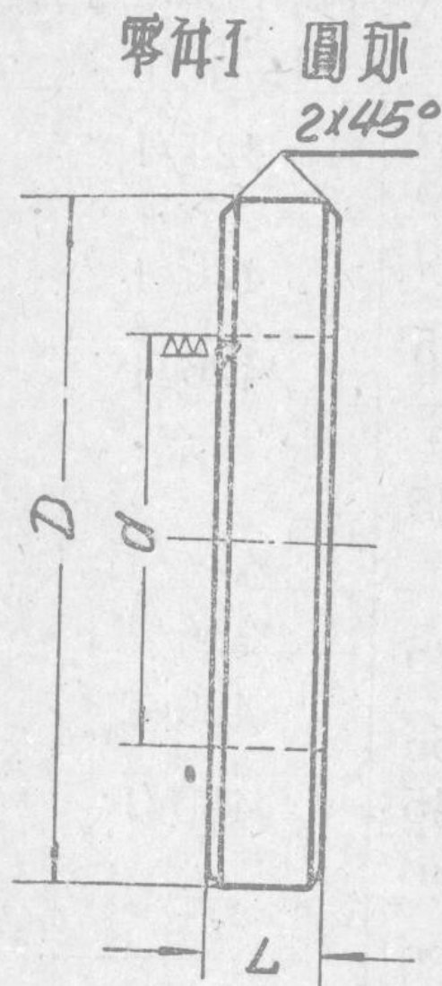
圓 环 的 图 例 符 号 d=28和D=79MM 78531—401/1
