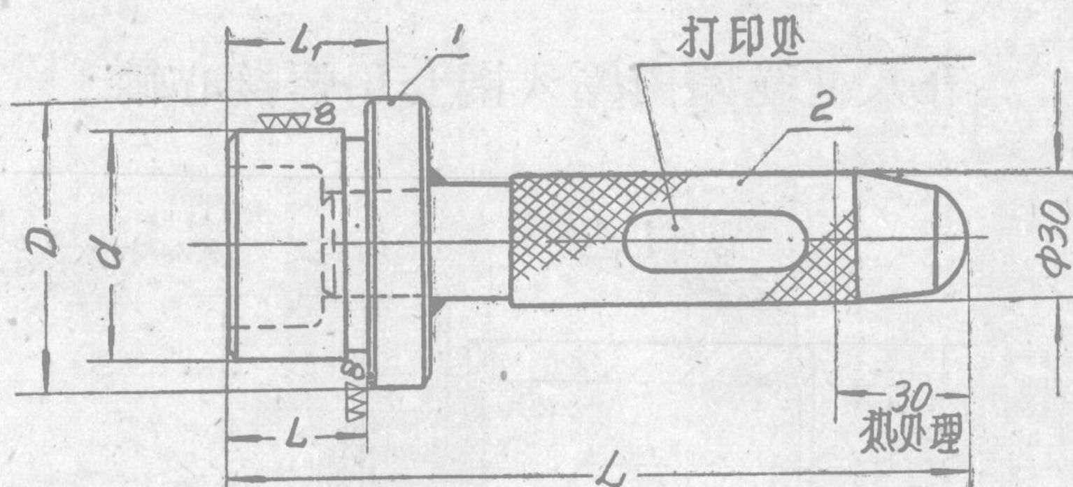
心 軸 的 图 例 符 号 d=49.5 和 L=30 MM 78531—101 MM
