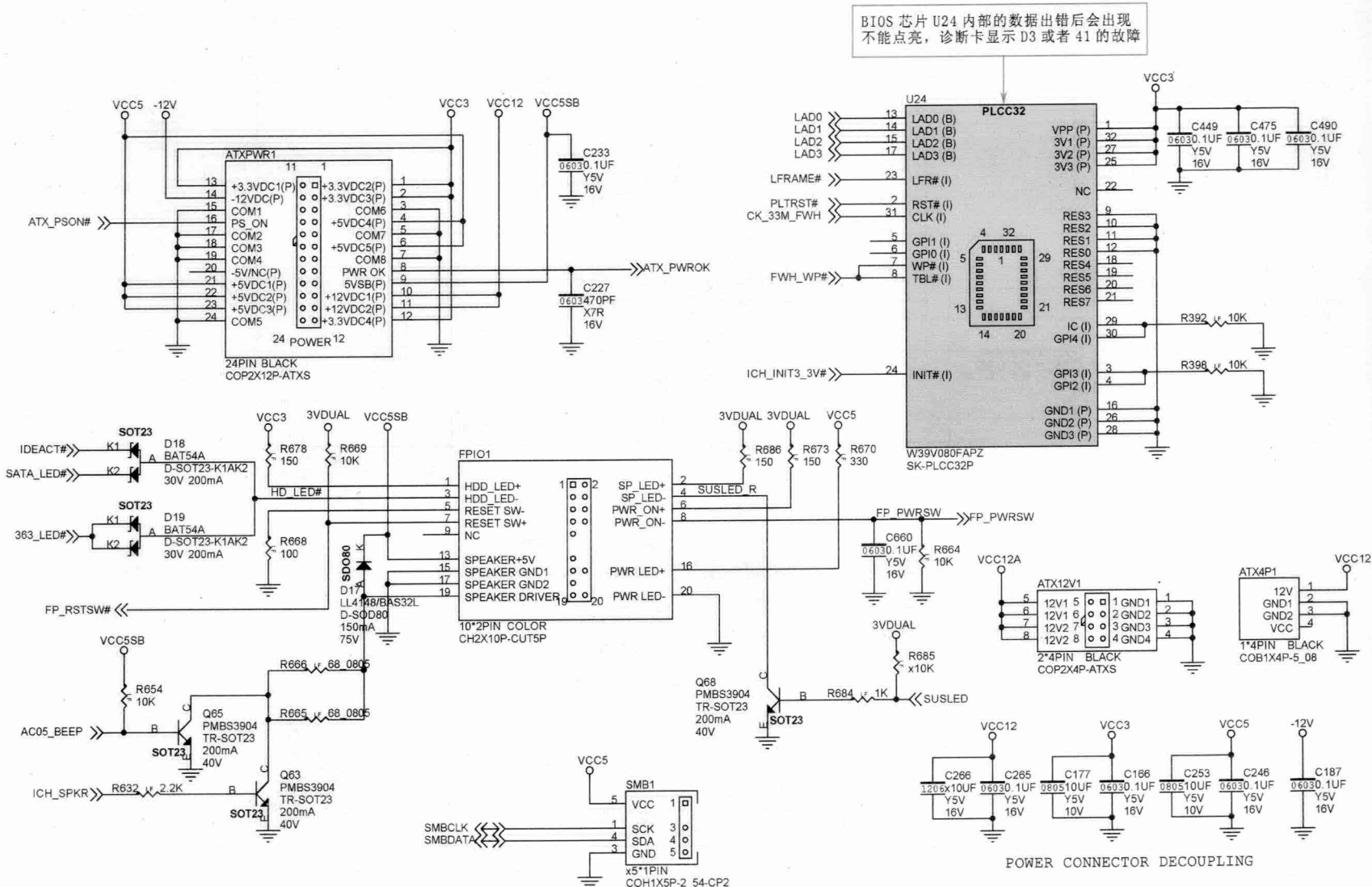
ABIT AB9 QuadGT前面板接口电路/BIOS电路维修图解
