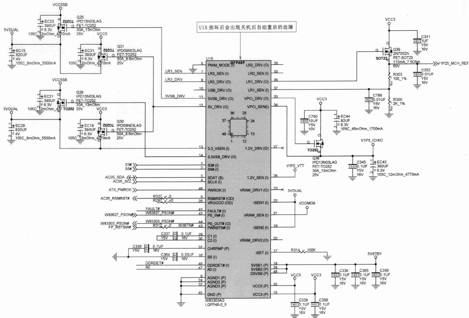
ABIT AB9 QuadGT 供电控制电路维修图解
