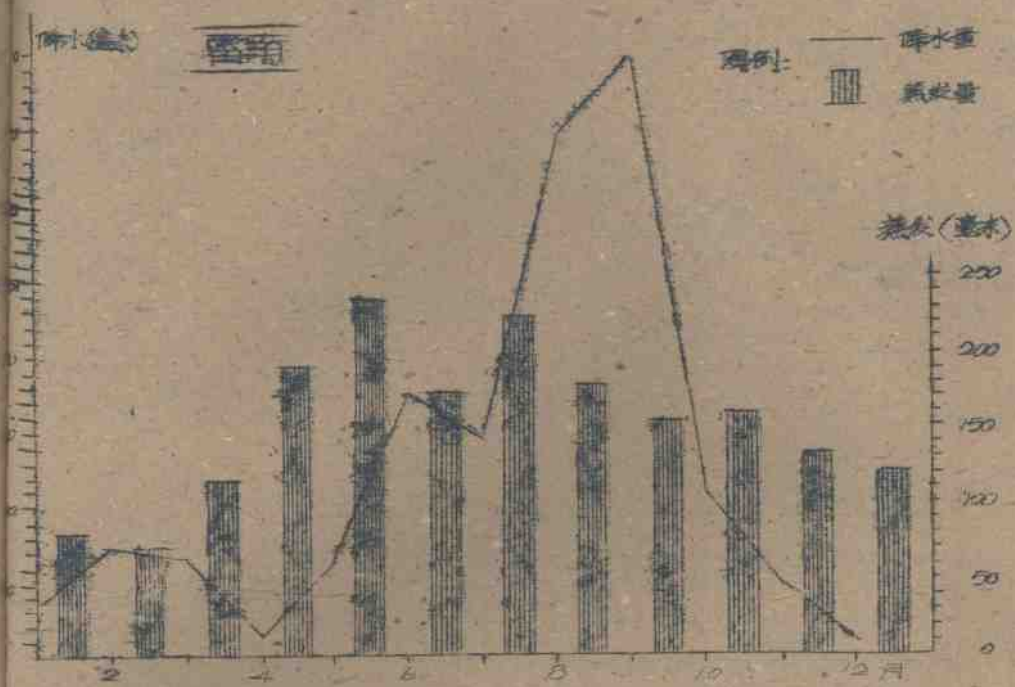
1957-1958年逐月平均降水量、蒸发量分布图
