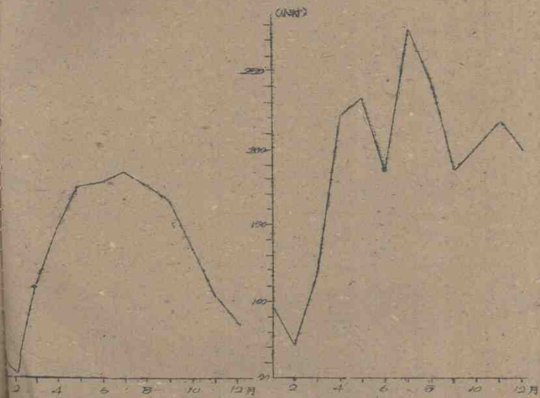
1957-1958年逐月平均气温分布图
