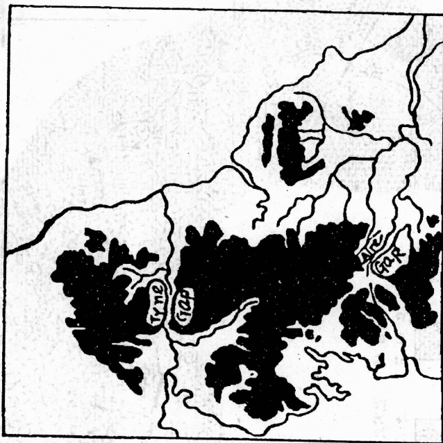
(附圖二) 北部英格蘭之景圖 以示泰尼(Tymel)與愛瑛(Aide)兩狹隘及功開府(Yorkshire)之特性。○黑色區域高六百尺。
