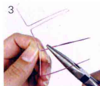
3. 将相邻两个“U”形的铁丝如图拧合。
