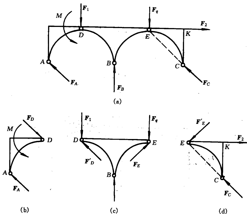
图 1-3 (错误的受力图)
