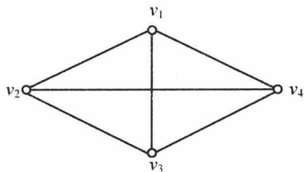
图 1.3 有四个顶点的图
