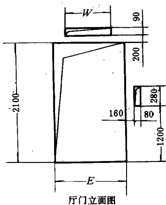
厅门立面图
