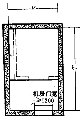
机房平面图
