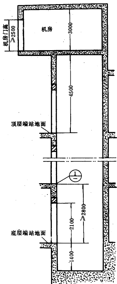
F—F 井道剖面图
