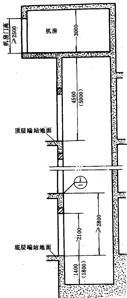
F-F 井道剖面图
