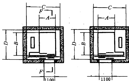
井道平面图(右开门)
