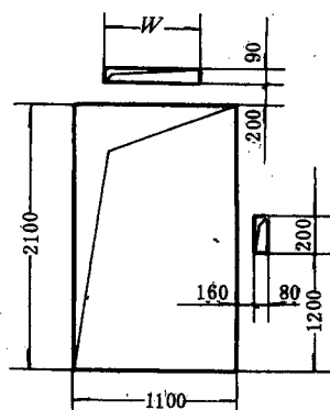
厅门立面图
