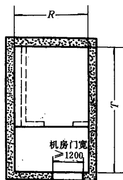
机房平面图
