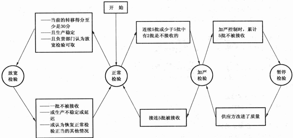
图 1 转移规则简图
