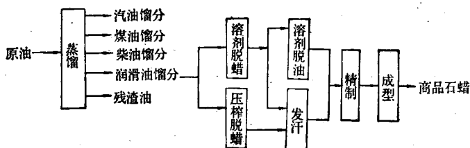
图 1 石蜡生产流程示意图
