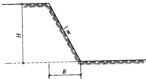
图 1-1 边坡坡度示意
