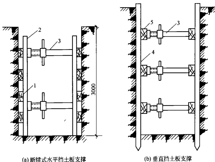
图 1-2 横撑式支撑
