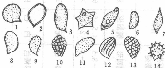
图6 孢子形状及表面特征
