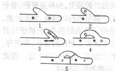
图1 锁状联合形成过程示意图
