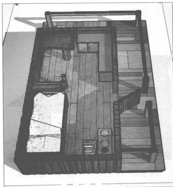
参考图 3：文中林间木屋一楼横截面 3D 示意图 (已标明窗户位置及大致高度)
