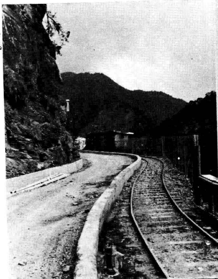
正施工中的茶華攔沙壩
