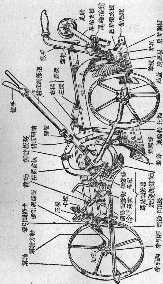
圖 1 雙輪雙鏵犁的構造
