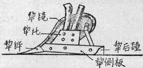
图2 犁头的构造
