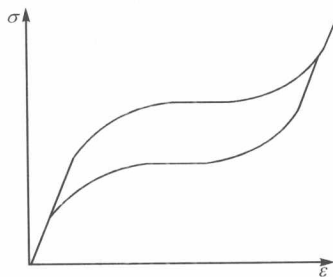
图 1.6 超弹性的应力-应变示意图
