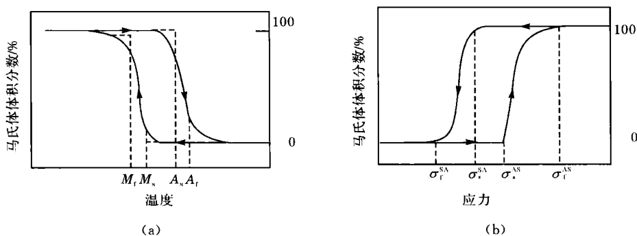
图 1.2 (a) 温度和(b) 应力诱发马氏体相变示意图
