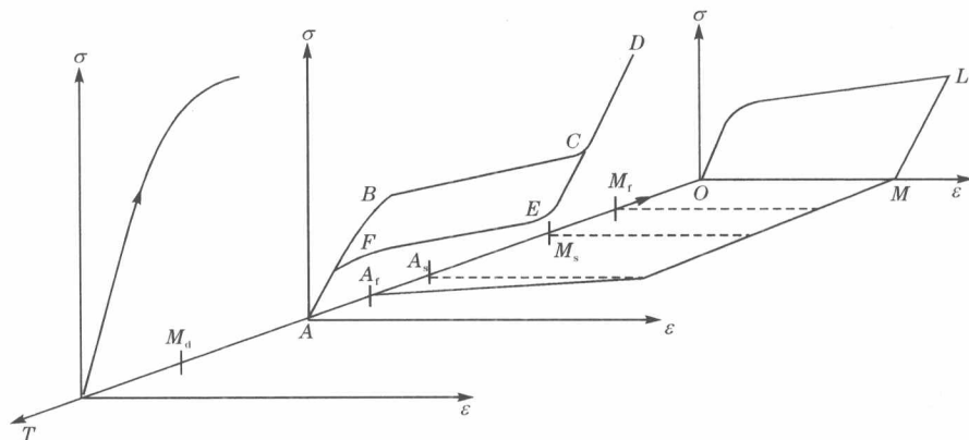
图 1.8 形状记忆合金在不同温度下的力学行为
