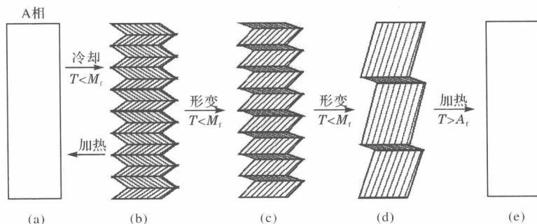
图 1.5 形状记忆效应的变形过程图
