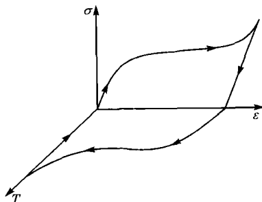
图 1.3 形状记忆效应的应力-应变-温度示意图
