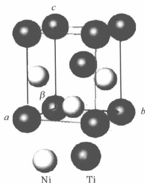
图 1.1 NiTi 形状记忆合金 B19' 马氏体的晶体结构
