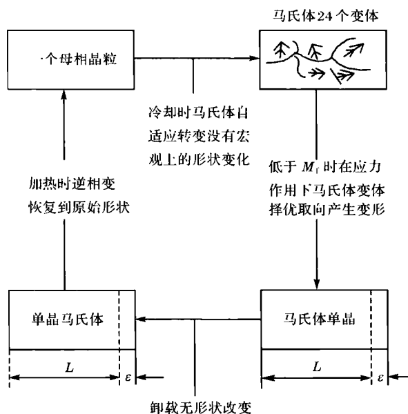
图 1.4 形状记忆效应原理示意图
