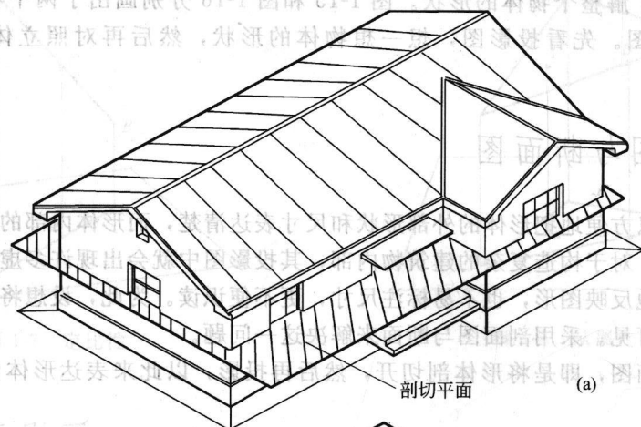
图 1-19 剖面图的表示方法
