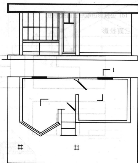
(b) 1-1 剖面平面图
