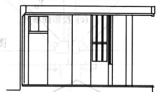
(c) 1-1 剖面立面图
