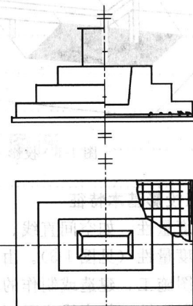
图 1-13 钢筋混凝土独立基础两面投影
