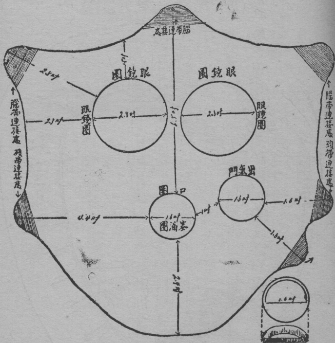
第三圖 面具之平面圖
