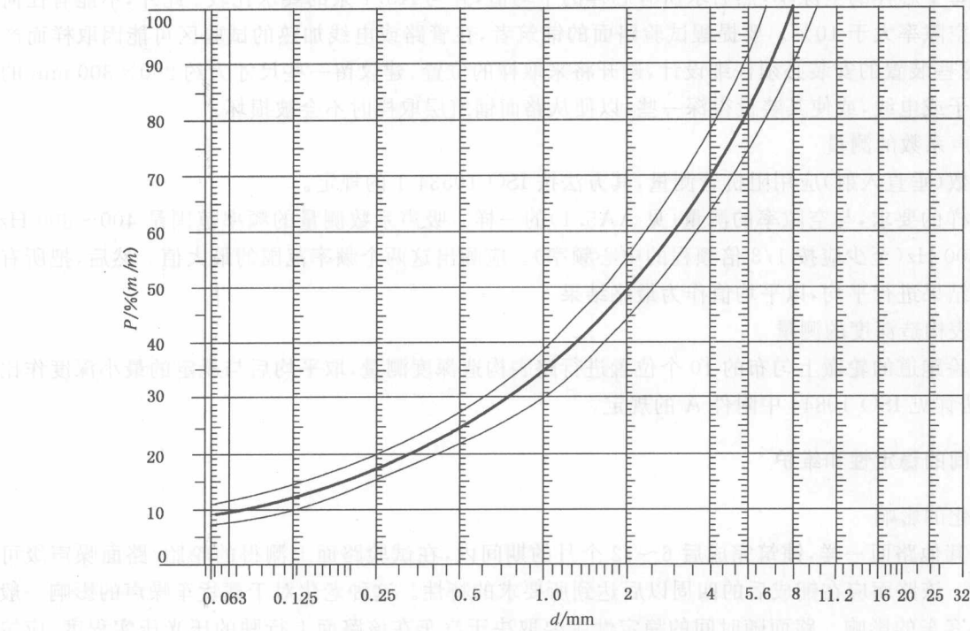
图 AA1 沥青混合料中石子级配曲线
