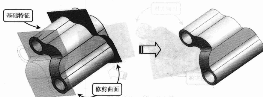
图 1-12 修剪法创建实体
