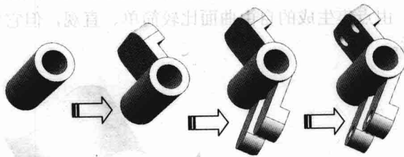
图 1-10 积木法创建三维实体
