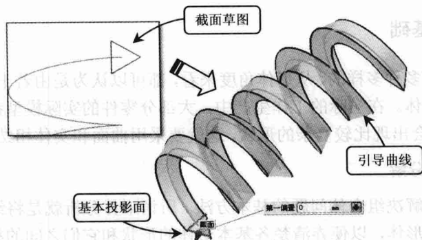
图 1-4 扫掠体截面生成实体
