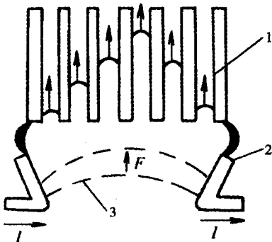
图 1-8 栅片灭弧
