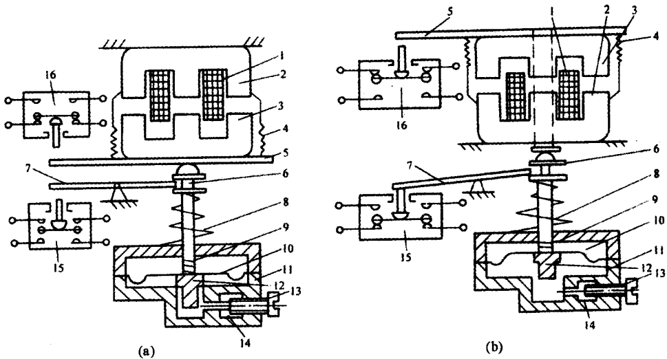
图 1-14 JS7-A 系列时间继电器
