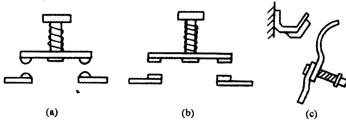
图 1-3 触点的结构形式
