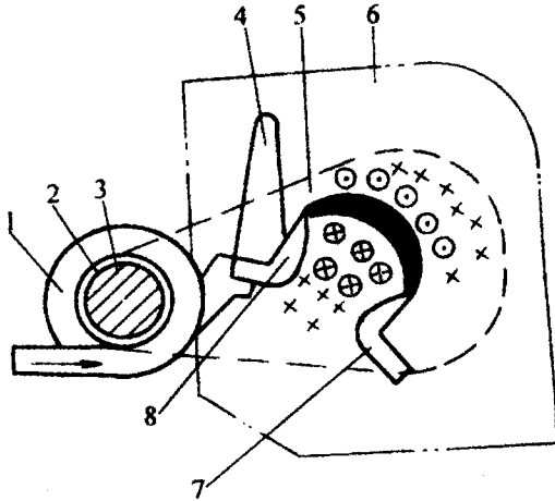
图 1-6 磁吹灭弧
