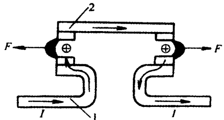
图 1-5 电动力灭弧
