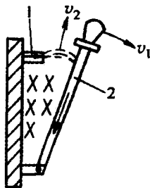
图 1-4 机械力灭弧
