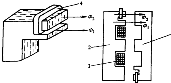
图 1-2 交流电磁铁的短路环 1—衔铁;2—铁芯;3—线圈;4—短路环
