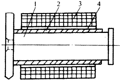
图 1-13 带有阻尼铜套的铁芯结构图
