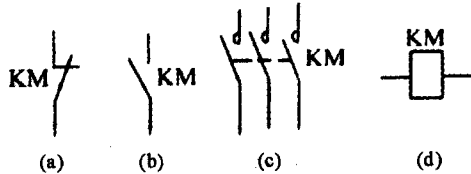
图 1-11 接触器的文字与图形符号
