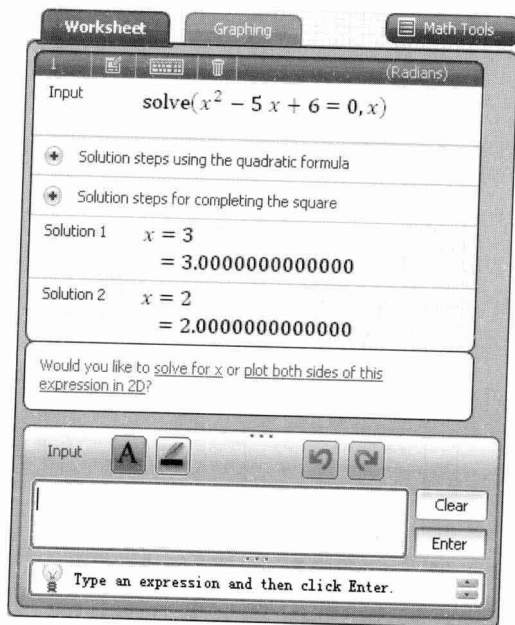
图 1.2 用解方程函数 solve 求解方程或方程组
