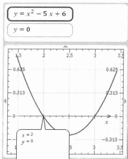
图 1.4 用图像法求解方程或方程组
