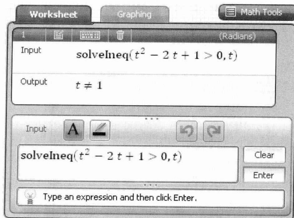
图 1.6 用解不等式方程函数 solveIneq 求解不等式方程
