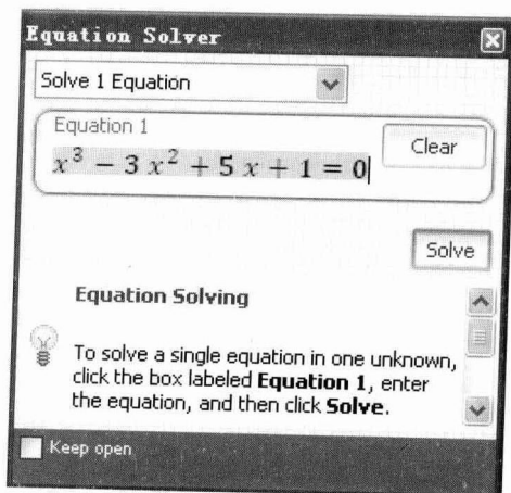
图 1.1 用解方程工具求解方程或方程组
