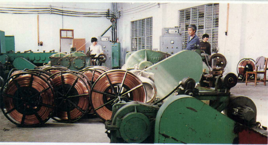
◀ 县电线厂拉丝车间
