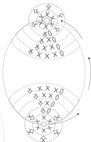
提手两端小球钩制针法图
