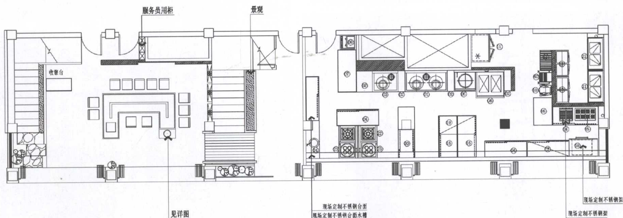
○ 一层平面布置图
