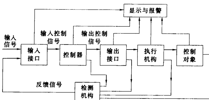
图 2-4 典型顺序控制系统的结构框图
