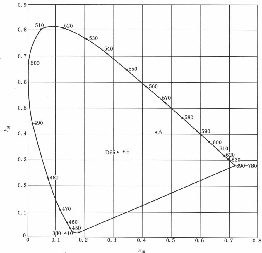
图 2 CIE1964 标准色度系统色品图
