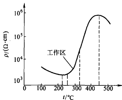
图 1-3 PTC 电热元件的电阻—温度特性
