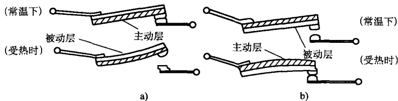
图 1-6 双金属片的结构 a) 常闭触点型 b) 常开触点型
