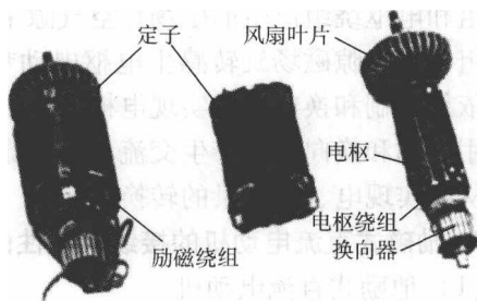
图 1-15 励磁式直流电动机的结构
