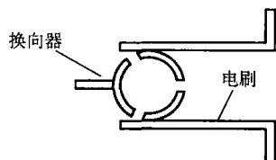
图 1-13 永磁式电动机的电刷
