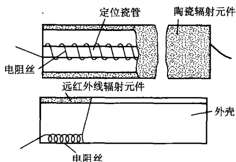
图 1-5 板状远红外线辐射元件
