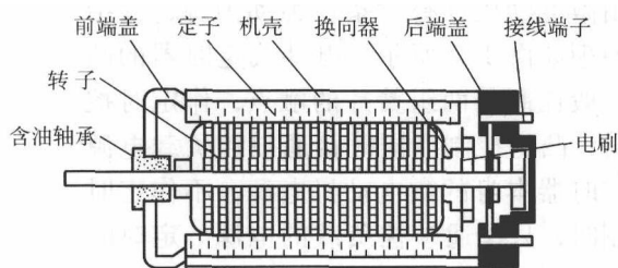
图 1-11 永磁式电动机结构
