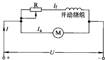
图 1-20 并励式直流电动机的接线
