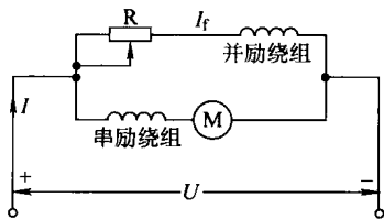
图 1-22 复励直流电动机的接线
