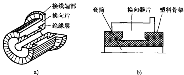
图 1-17 换向器的结构
