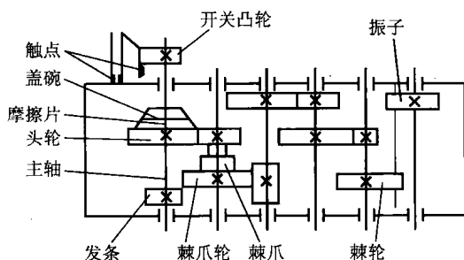
图 1-8 机械式定时器结构原理
