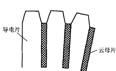
图 1-16 导电片和云母片结构
