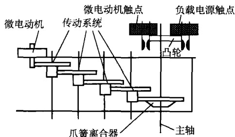
图 1-9 电动式定时器结构原理
