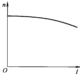
图 1-23 复励直流电动机电枢电流与转速的关系
