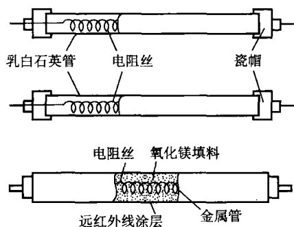
图 1-4 管状红外线辐射元件
