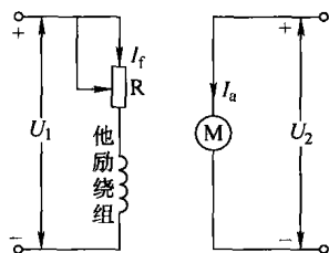
图 1-18 他励式直流电动机的接线
