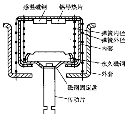
图 1-7 磁控式温控器
