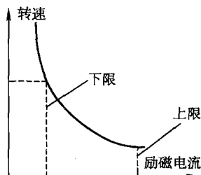
图 1-19 励磁电流与转速的关系
