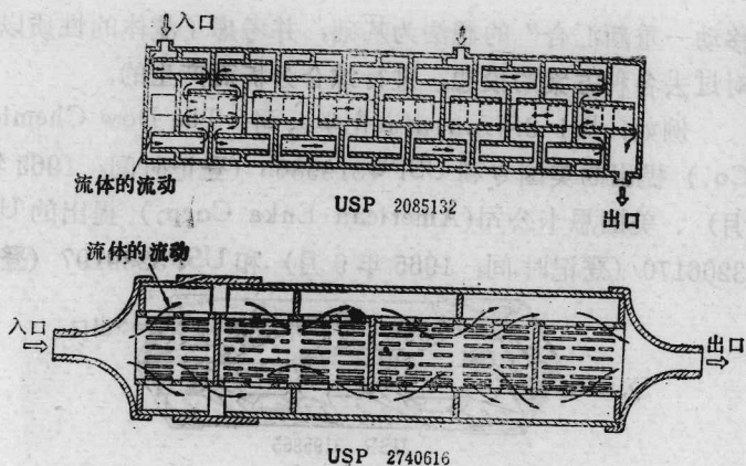
图1-1 静态混合器产生以前的流体管路结构体
