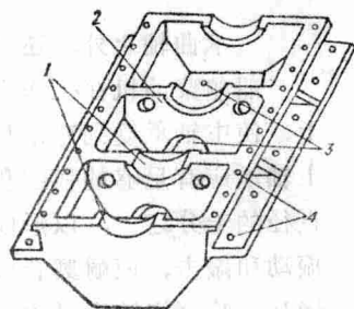
图2-2 柴油机机座 1-主轴承座；2-横隔板； 3-油孔；4-螺孔
