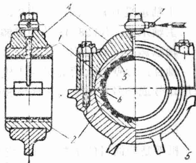
图2-4 正置式轴承 1-上轴瓦；2-下轴瓦；3-耐磨合金； 4-轴承盖；5-轴座；6-垫片；7-油管
