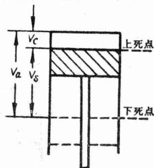
图1-3 气缸容积
