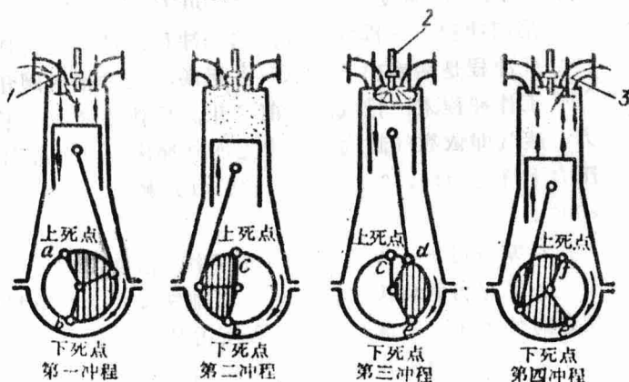
图1-4 四冲程柴油机工作原理图
