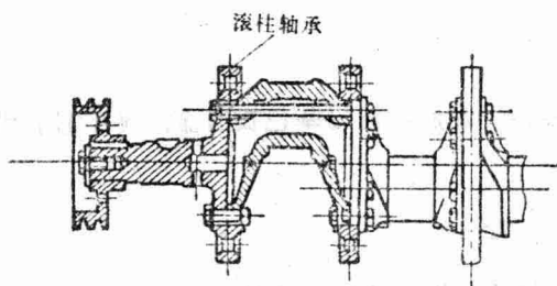
图2-3 滚柱轴承
