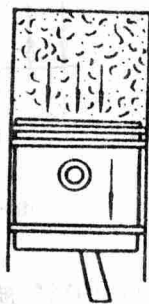
图1-1 燃料在气缸内爆炸做功示意图
