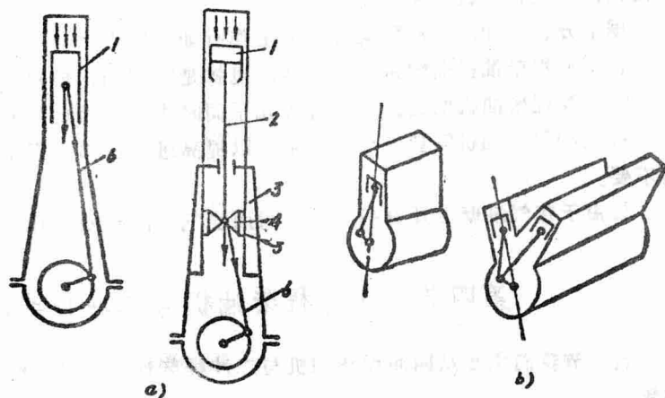
图1-6 气缸排列型式
