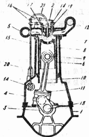
图1-2 四冲程柴油机的主要部件
