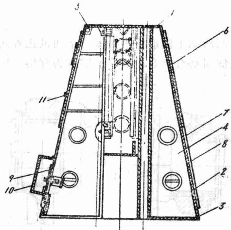
图2-6 A字型机架
