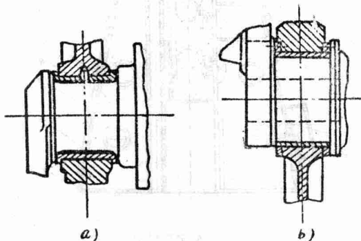
图2-5 定位轴承 a)翻边；b)平
