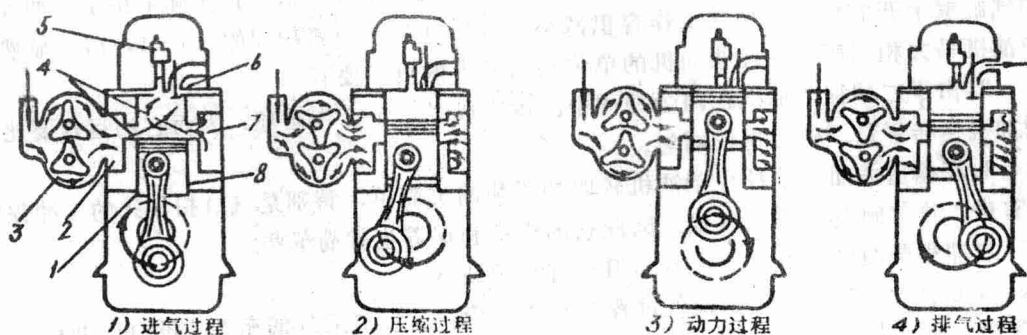
图1-5 二冲程柴油机工作原理图
