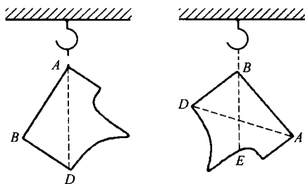
图 1-4 悬挂法求形状不规则物体的重心
