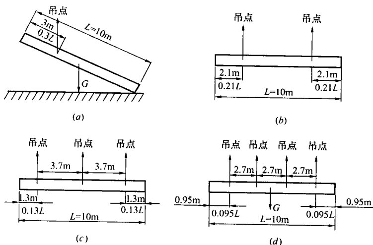
图 1-5 吊点位置选择示意图
