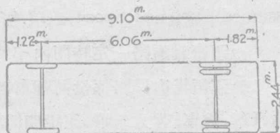
(b) 設計貨車或公共汽車尺寸
