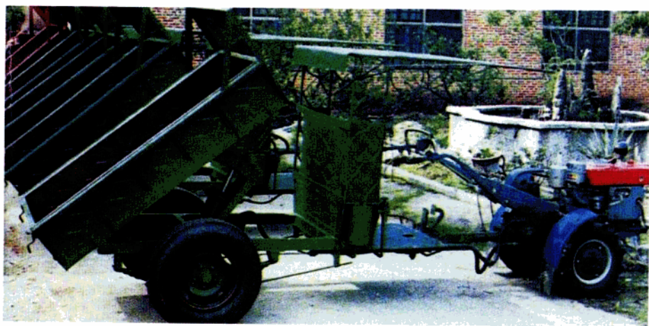
► 西湾矿务局 (原西湾煤矿) 机修厂生产液 压自卸拖斗， 1989 年获自治 区百花奖。
