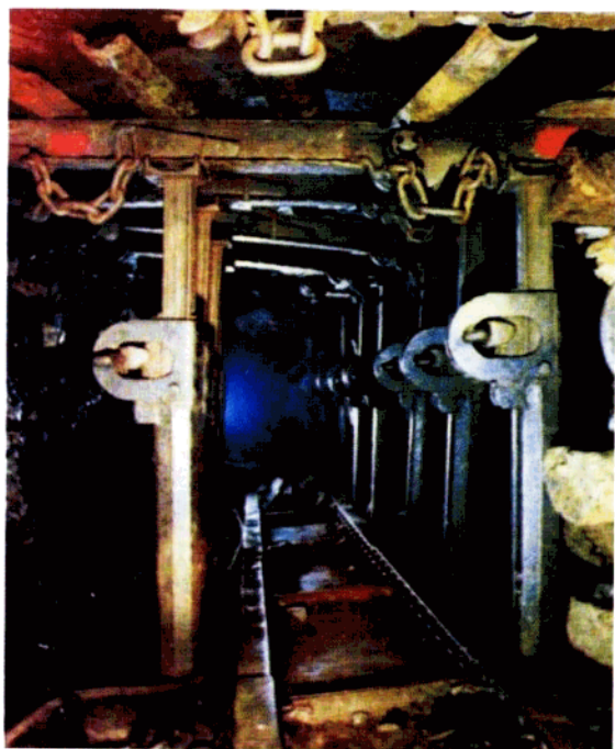
▲1989年右江矿务局质量标准化采煤工作面。
