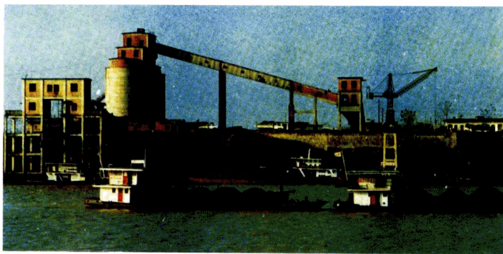
▲ 1979 年建成投入运营的那龙矿务局右江装煤码头。
