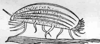
第四圖 原狀生動物之名為 Euploes harpa 者
