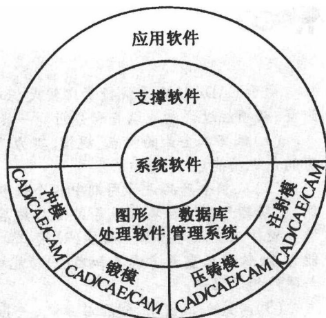
图 1-4 模具 CAD/CAE/CAM 系统软件层次图
