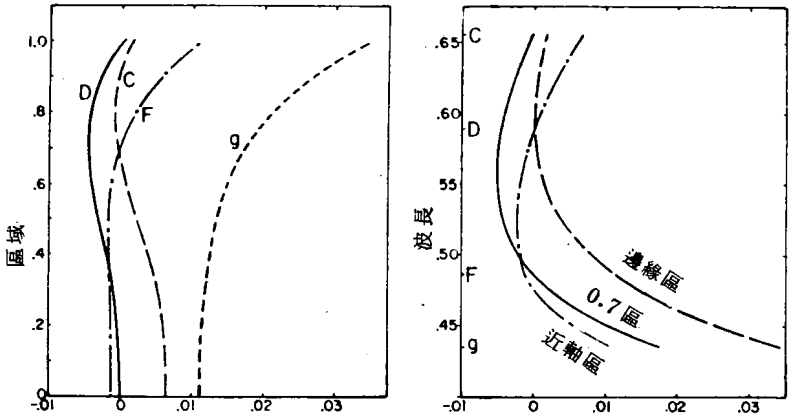
圖 3 消色雙透鏡的球面色差
