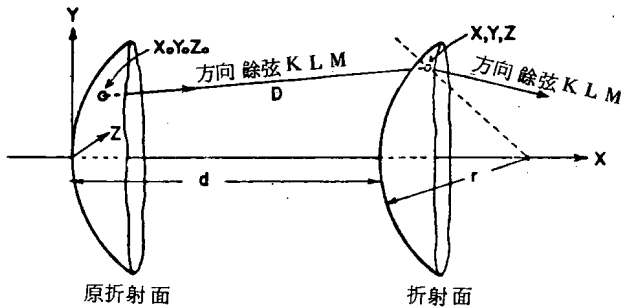
圖 2 斜射線自折射面轉移到另一折射面的情形
