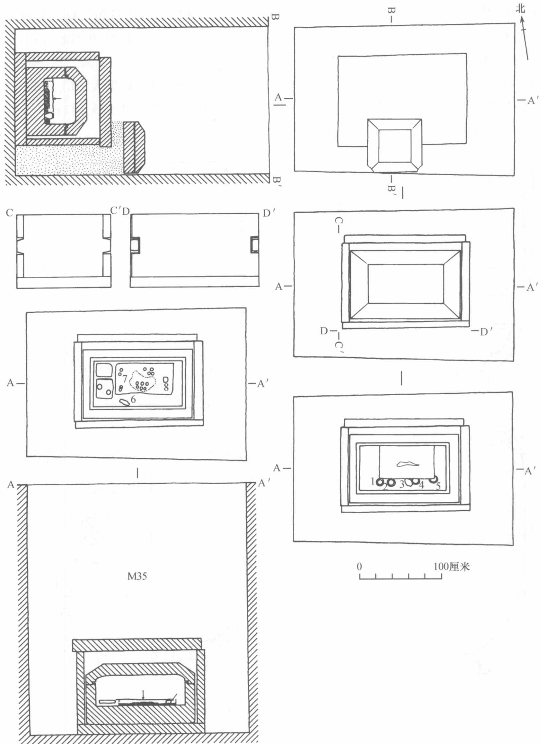
图三 M35 平、剖面图
