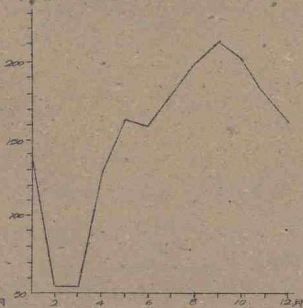
1956—1957年逐月平均日照时数分布图
