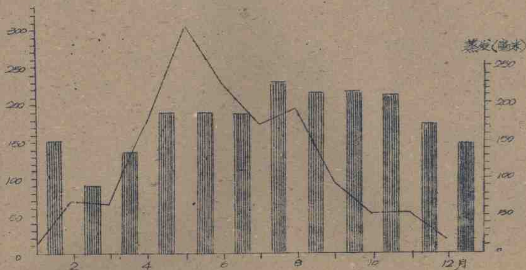
1956—1957年逐月平均降水量、蒸发量分布图
