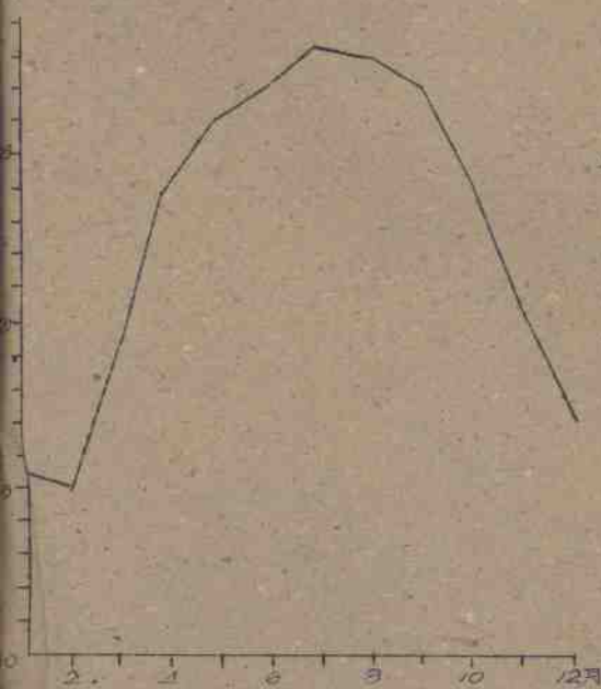
1956—1957年逐月平均气温分布图
