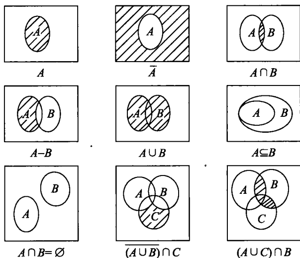
图 1 Venn 图
